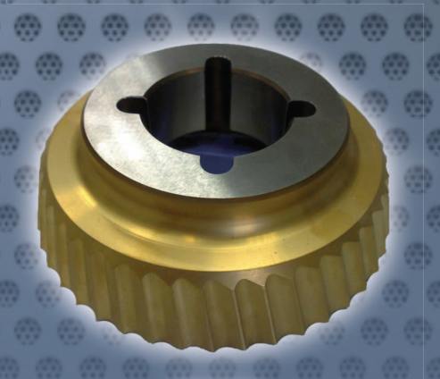
製品番号 Art. Nr. 2136 - cutter UZ15
